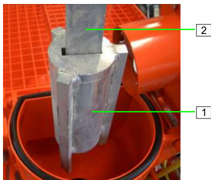
Abb. 77: Mischrohrreiniger einsetzen
