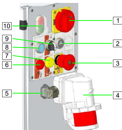
Abb. 13: Baugruppe Schaltschrank
