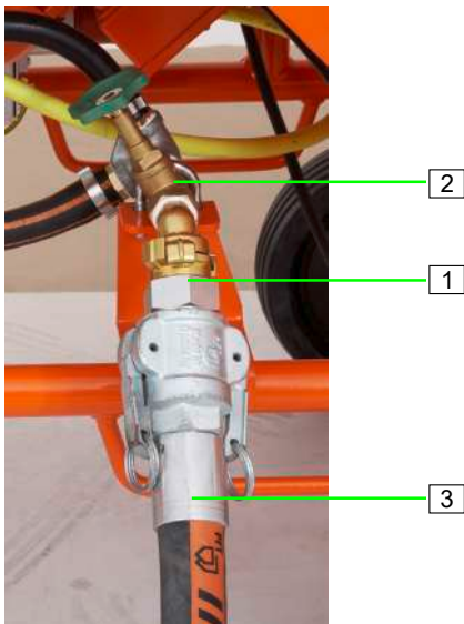
Abb. 41: Mörtelschlauch vorbereiten
