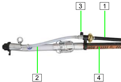
Abb. 45: Spritzgerät
