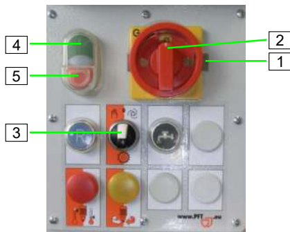
Abb. 85: Maschine wieder einschalten
