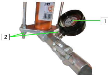
Abb. 65: Mörteldruck überprüfen und ablassen
