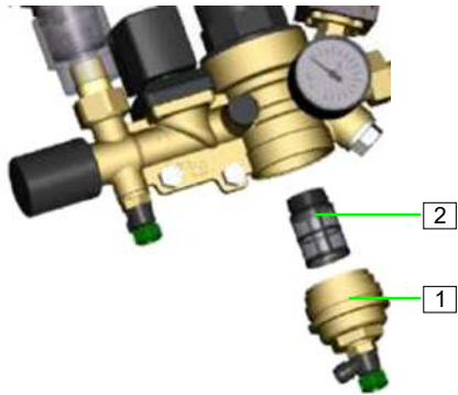
Abb. 91: Schmutzfängersieb
