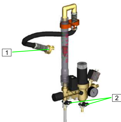
Abb. 67: Wasserzufuhr trennen
