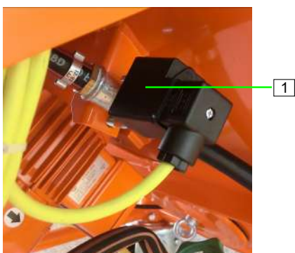
Abb. 93: Druckschalter Luft
