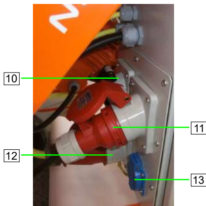
Abb. 12: Baugruppe Schaltschrank
