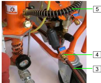
Abb. 33: Wasser anschließen
