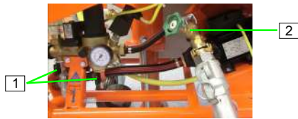
Abb. 32: Ablasshähne schließen
