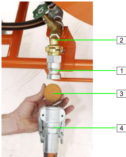
Abb. 73: Mörtelschlauch reinigen
