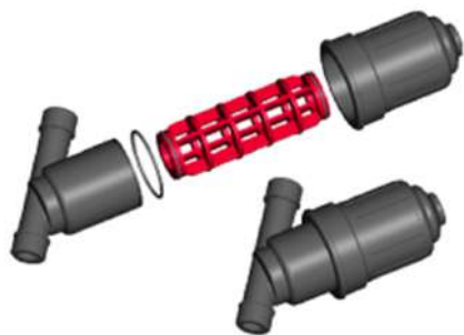
Abb. 68: Schmutzfänger
