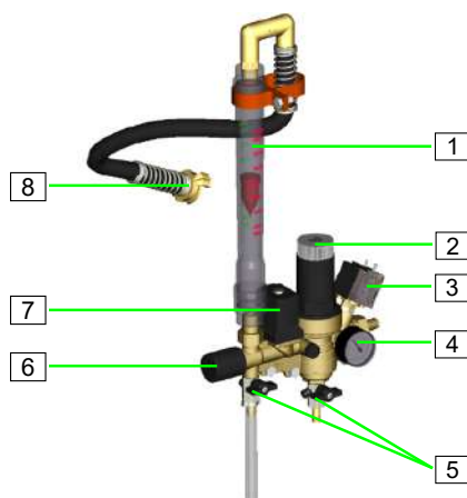
Abb. 15: Baugruppe Wasserarmatur
