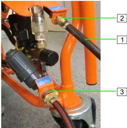
Abb. 69: Luftschauch anschließen
