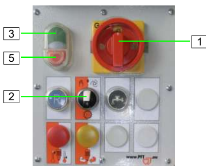
Abb. 54: Maschine einschalten
