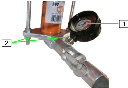
Abb. 83: Mörteldruck überprüfen und ablassen
