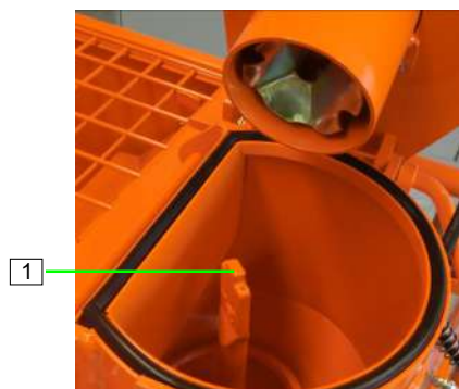
Abb. 76: Motorkippflansch öffnen
