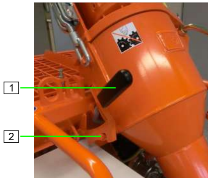
Abb. 95: Mischrohr hochklappen
