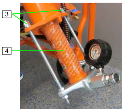
Abb. 96: Pumpe wechseln
